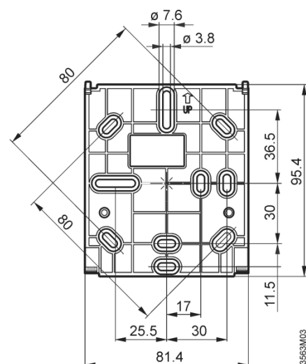
Bodenplatte
