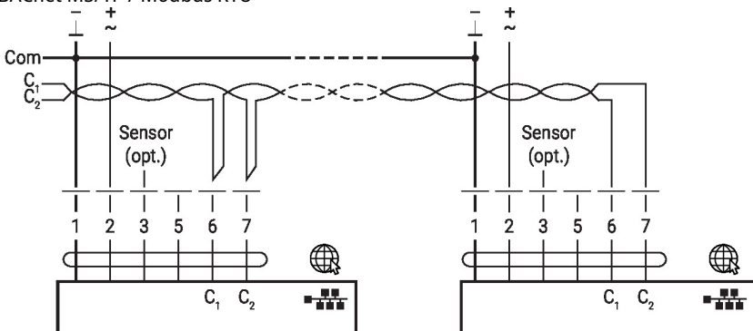
BACnet MS/TP / Modbus RTU
