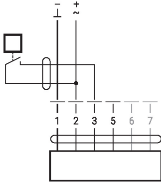
Raccordement avec contact de commutation
