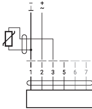
Raccordement avec capteur passif
