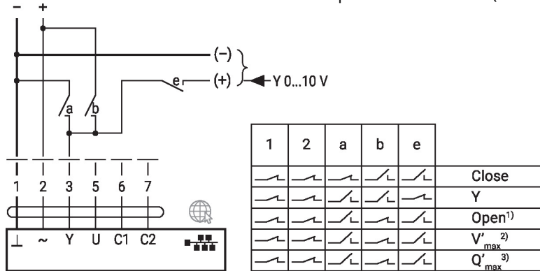
Commande forcée et limitation avec alim. AC 24 V par des contacts relais (avec commande classique ou hybride)
