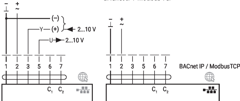
PoE avec BACnet IP/Modbus TCP
