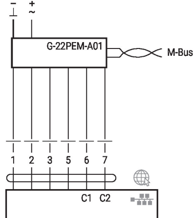
AC 230 V, tout-ou-rien
