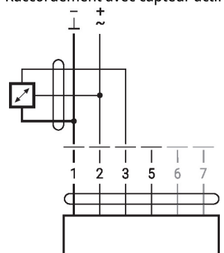
Raccordement avec capteur actif
