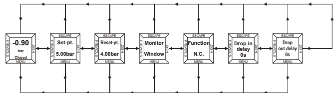
Abb. 3. DISPLAYBEREICH
