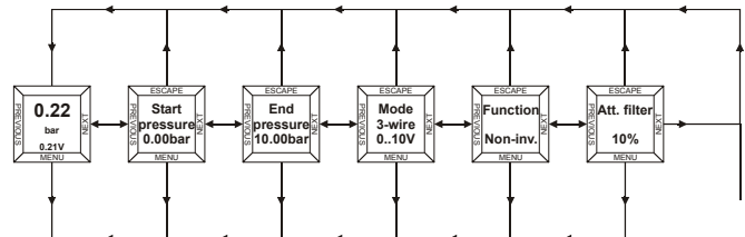
Abb. 12. DISPLAYBEREICH (Beispiel: SN 3-Leiter)
