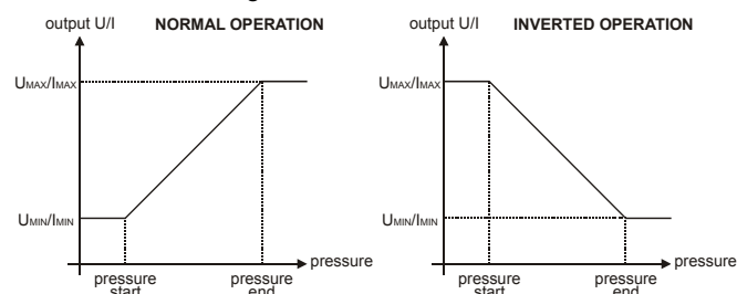
Abb. 15. SN Transmitter Ausgang (normal/invertiert)
