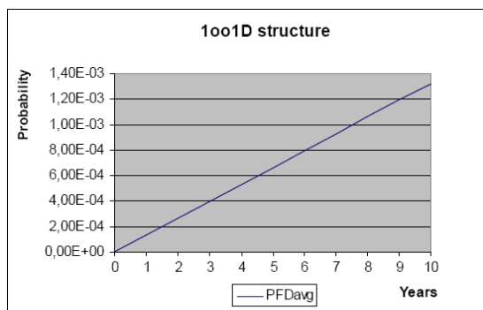
Abb. 17. Testintervalle und PFD avg
