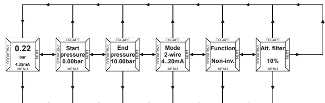
Abb. 11. DISPLAYBEREICH (Beispiel: SN 2-Leiter)
