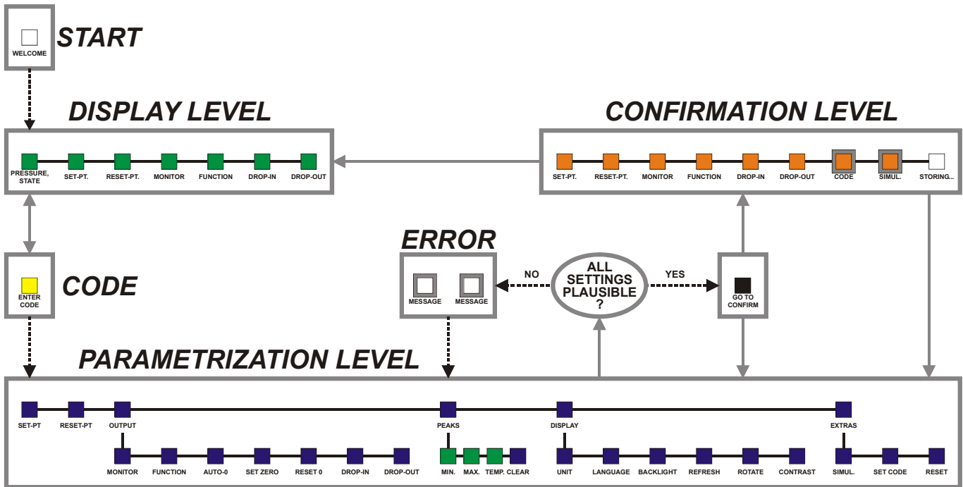
Abb. 1. Menünavigation - Übersicht (DCM)
