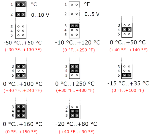
Abb.: (Messbereichs- und Offsettingstellung, Standardeinstellung: -50 °C..+50 °C | 0 K)
