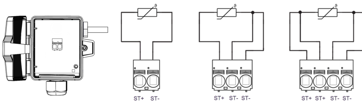
Abb.: (Anschlussbelegung passiver Sensor)
