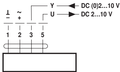
LRF24-SR
