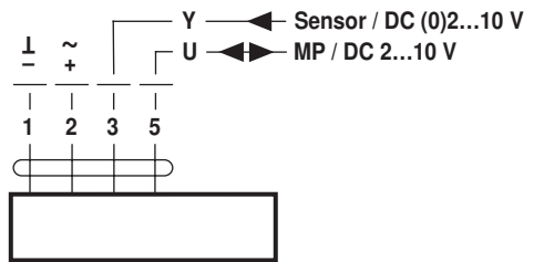
LRF24-MP (-O)
