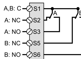
Abb. 10 Endlagenschalter (Nxx-SW2)
