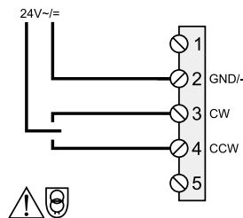
Abb. 7 N0524/N1024 (Dreipunktbetrieb)
