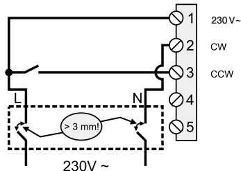
Abb. 9 N05230-2POS/N10230-2POS (Zweipunktbetrieb)
