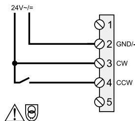
Abb. 8 N0524/N1024 (Zweipunktbetrieb)
